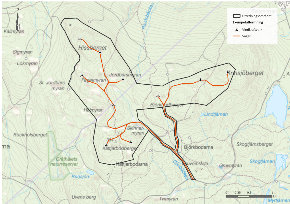
FIGUR 4 Exempel på utformning för Hissberget vindkraftpark.
